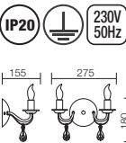
02-710 E14, 2 x max. 28W
