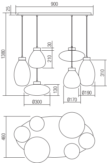
01-3212 Sand Black E27, 6 x max. 42W
