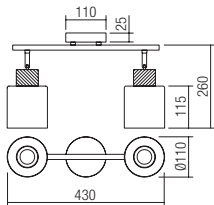
04-528 E27, 2 x max. 42W IP20 230V 50Hz
